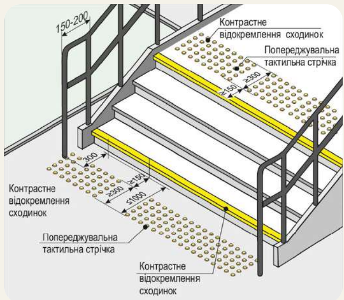
Рисунок 1.14. Облаштування сходинок
